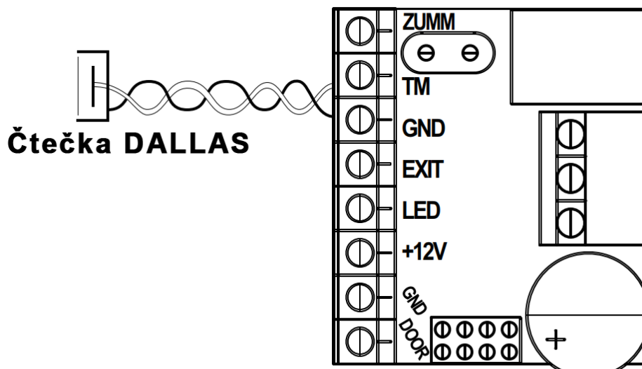
Obrázek 5: Připojení čtečky DALLAS
