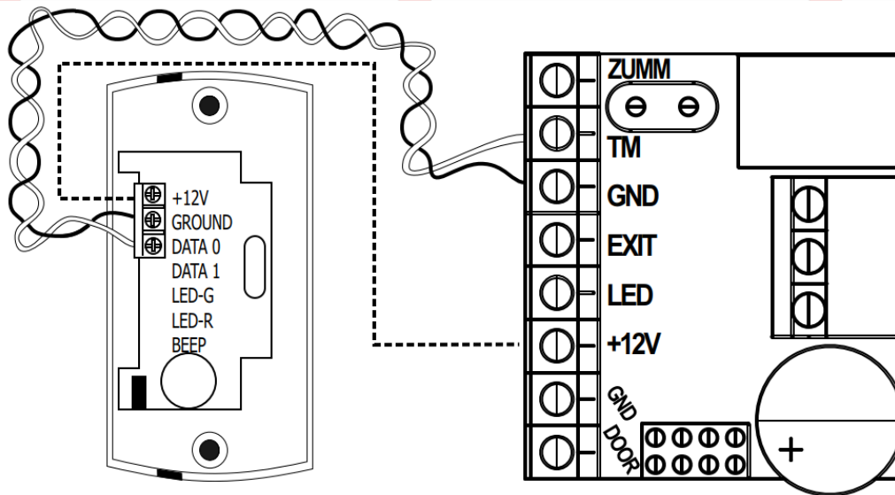
Obrázek 4: Připojení externí čtečky
