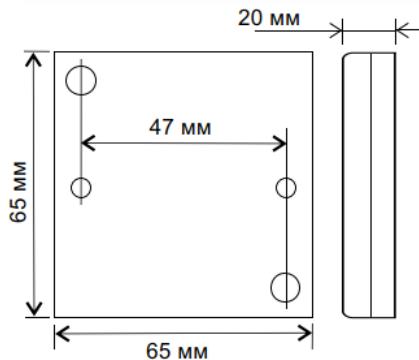
Obrázek 1: Rozměry pouzdra
