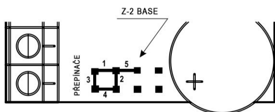
Obrázek 3: Pozice propojky
