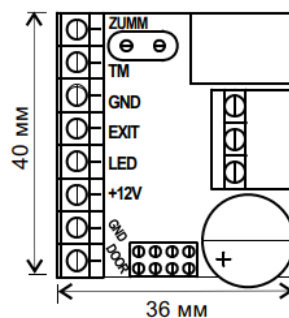
Obrázek 2: Rozměry plošného spoje PCB
