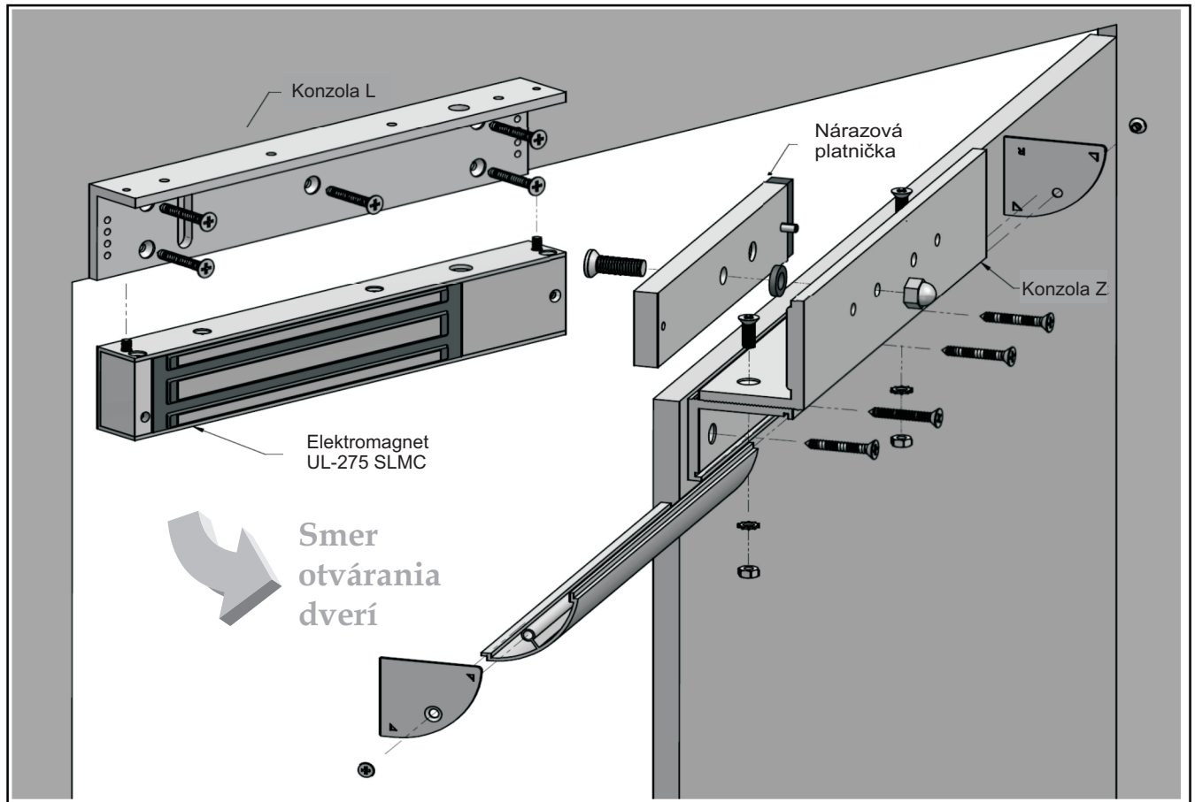
Obrázok 1. Schématický Pohľad
